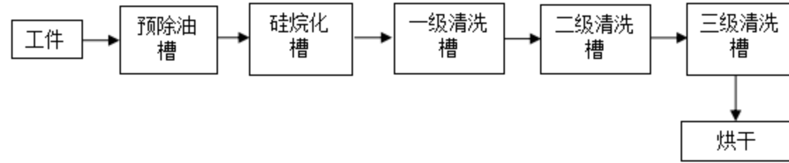
图 1 项目除油硅烷化清洗装置连接图
