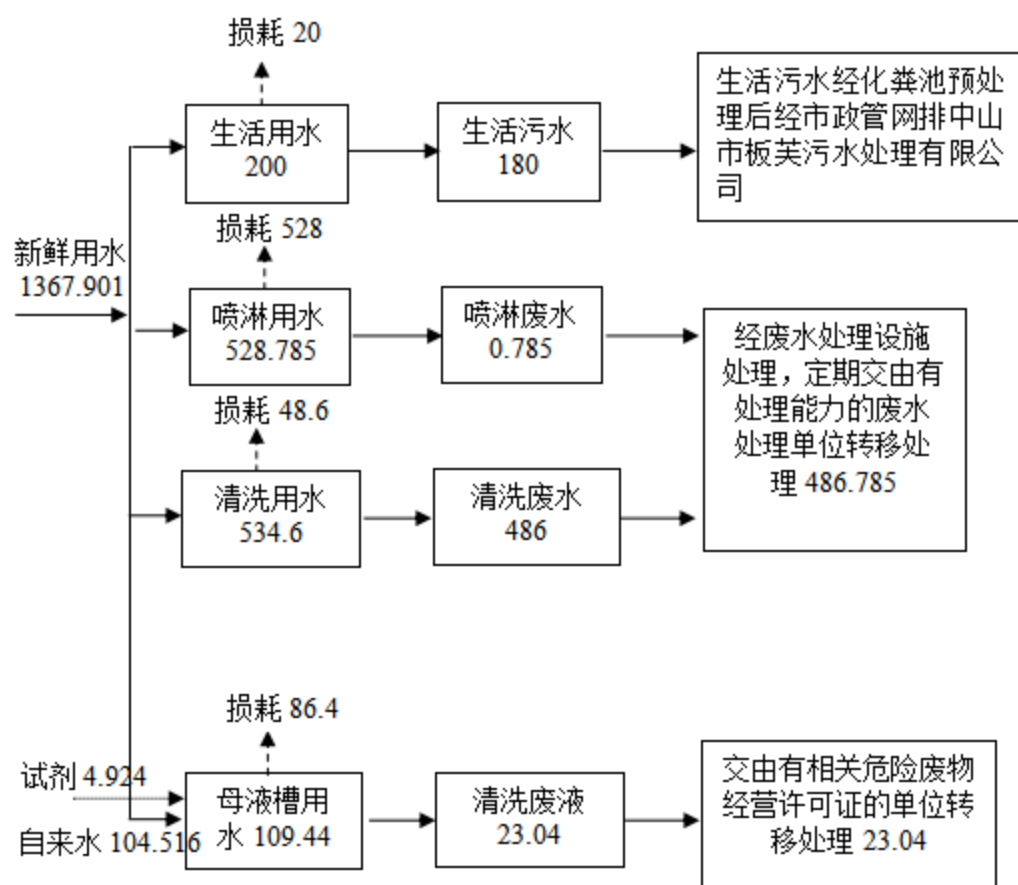
图3 水平衡图 (单位: t/a)
