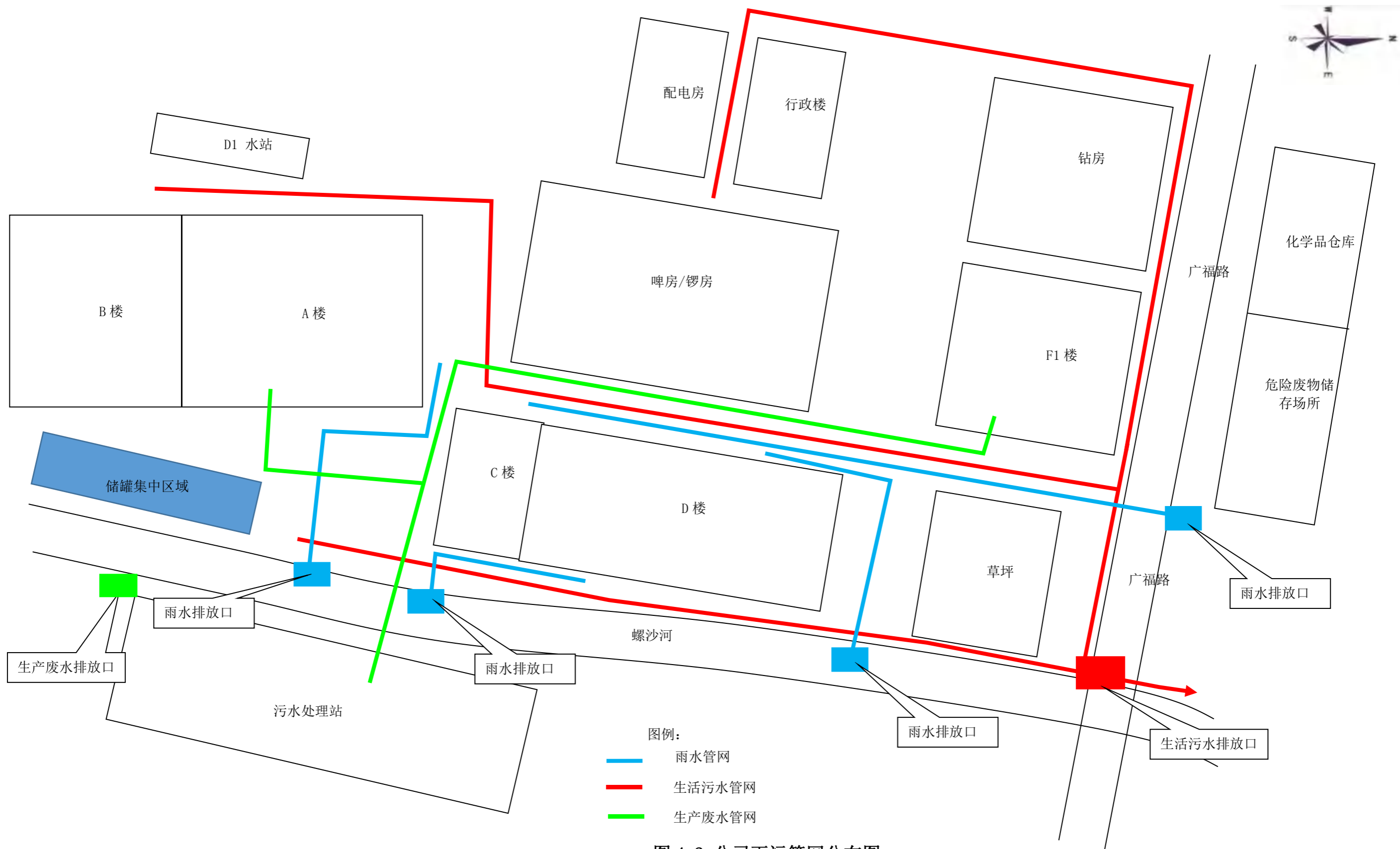
图 4-2 公司雨污管网分布图
