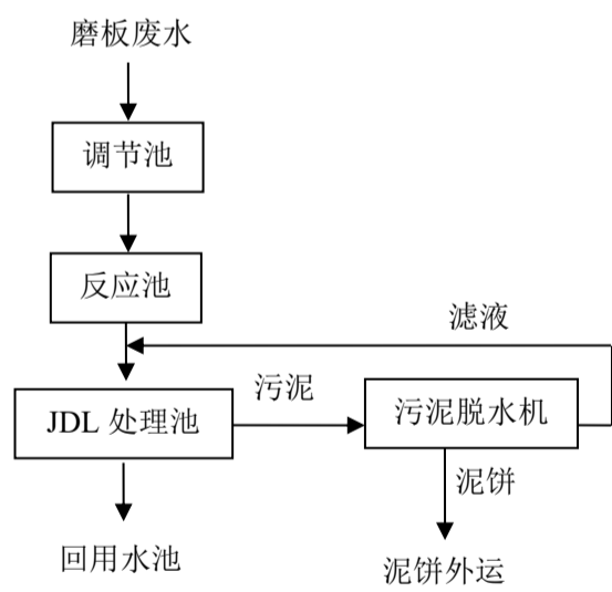
图 4-4-2 二期污水处理工艺流程图
