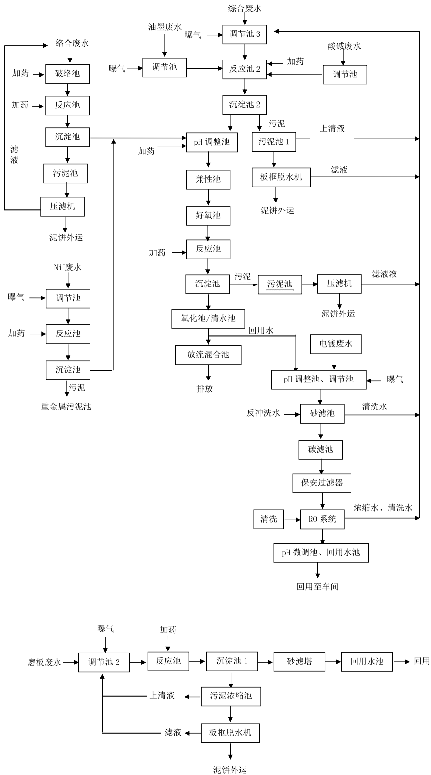
图4-4-1 一期废水工艺流程图
