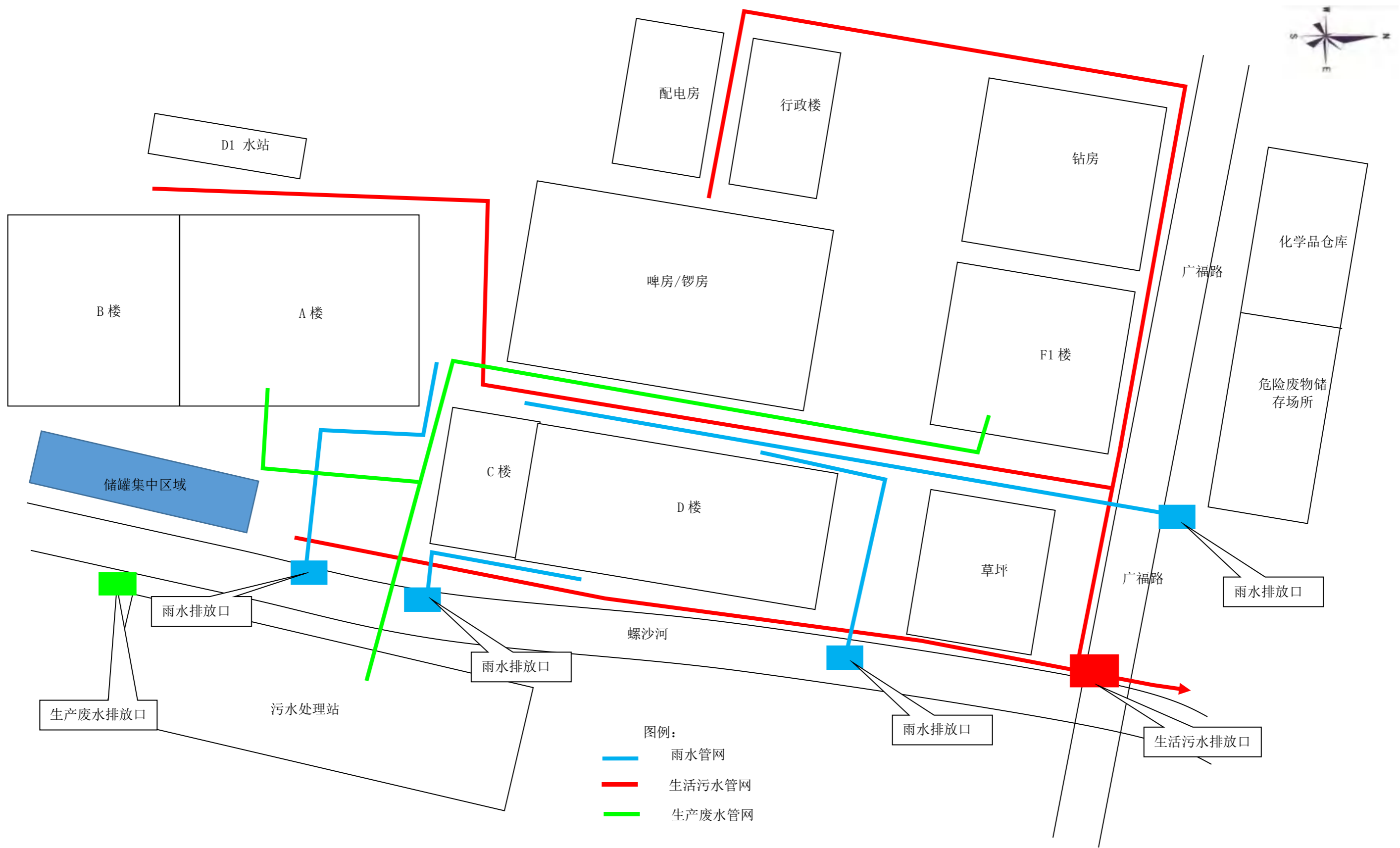
图 4-13 公司雨、原料管道管网分布
