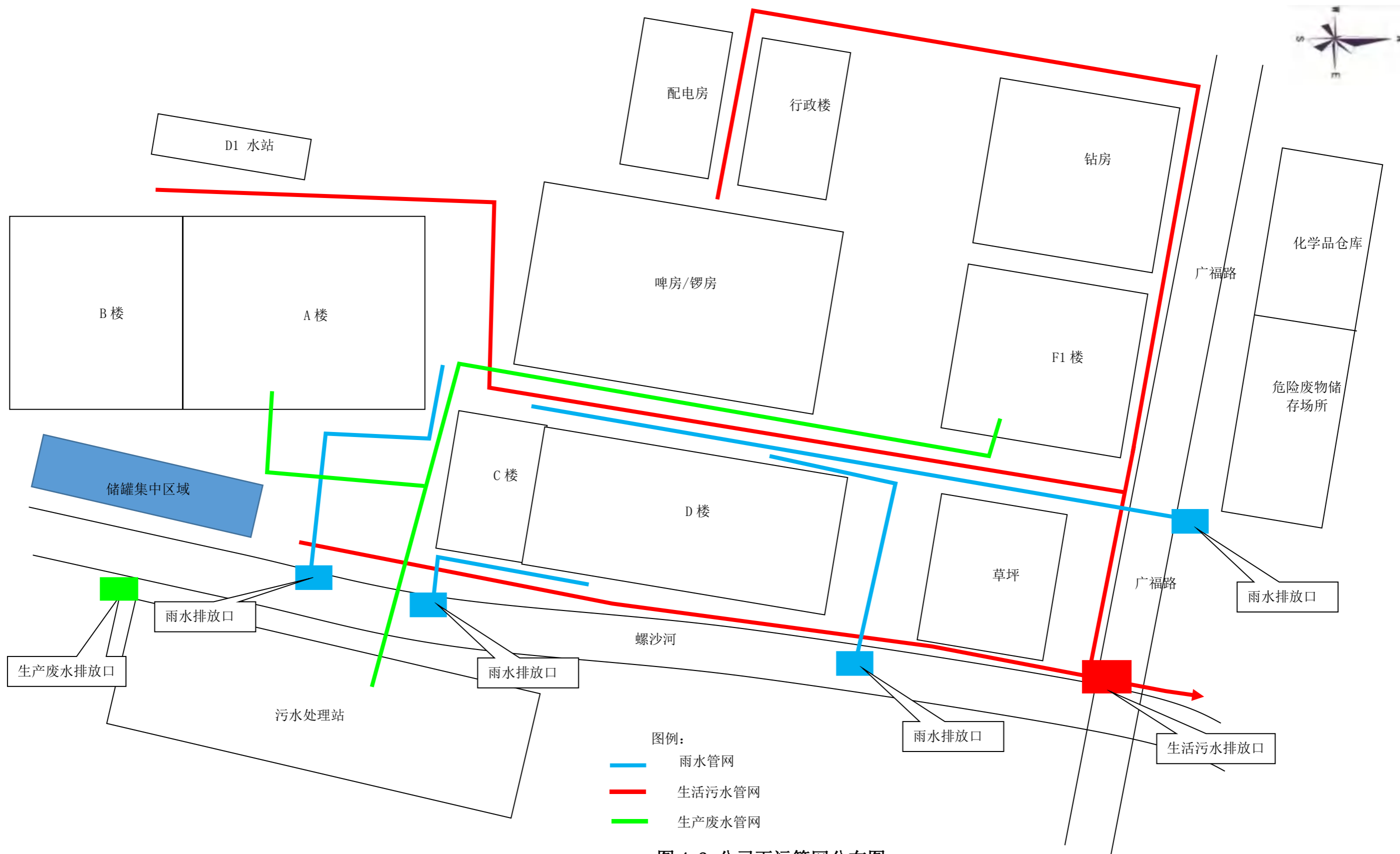
图 4-2 公司雨污管网分布图
