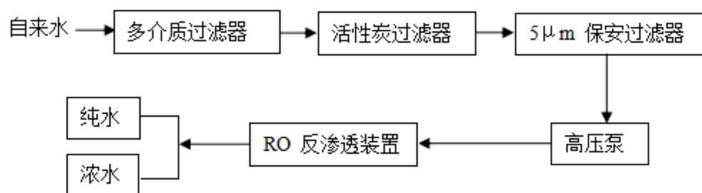
图 9 纯水制备工艺流程图
