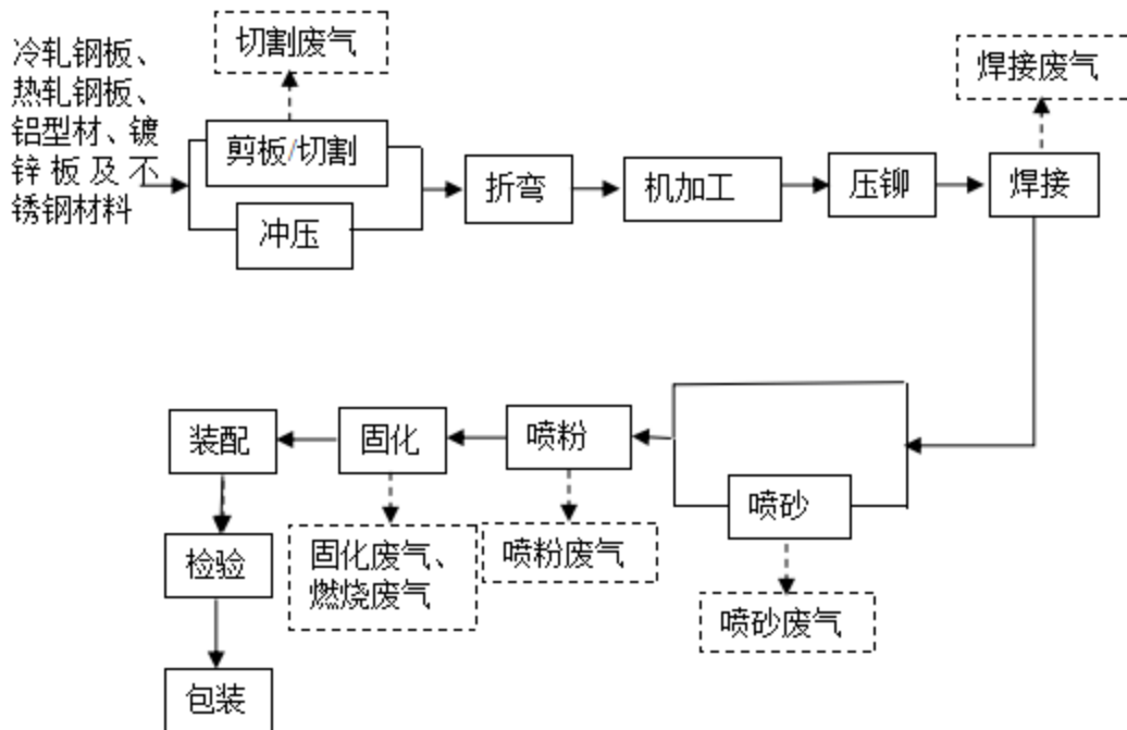
图3 总生产工艺流程图
