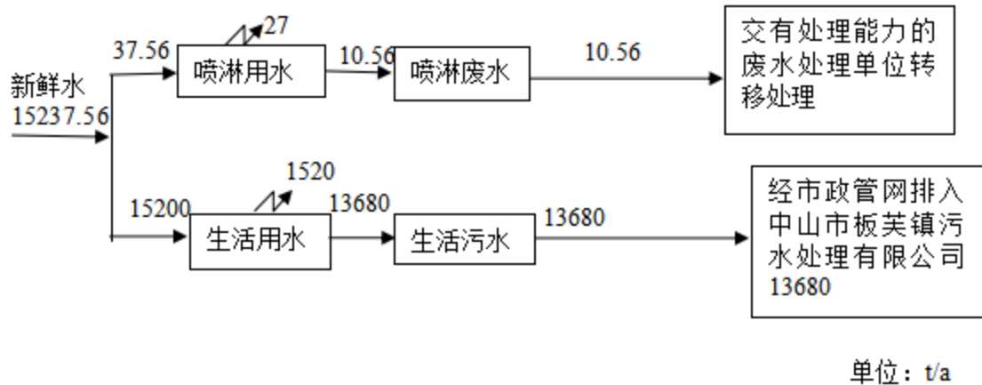
图 2 项目搬迁后水平衡图
