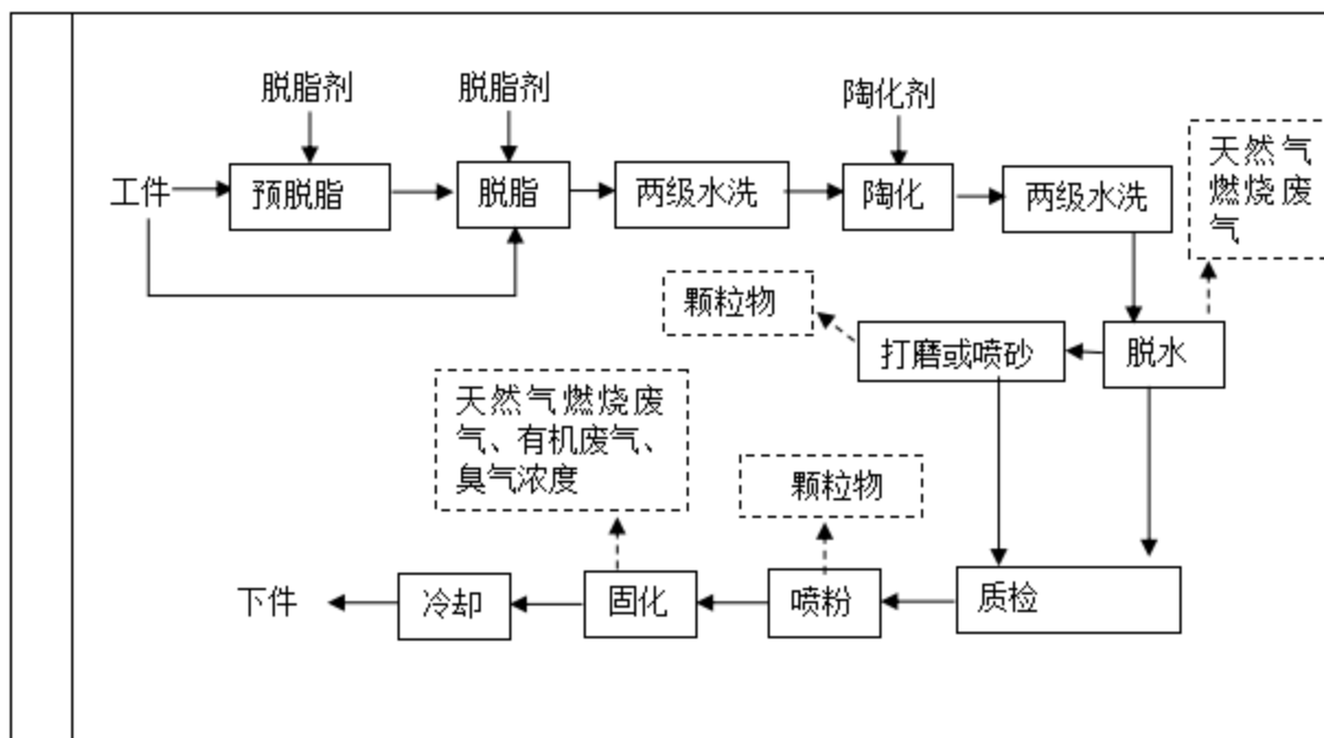
图 6 电梯轿厢整体集成系统等喷粉生产工艺流程图
