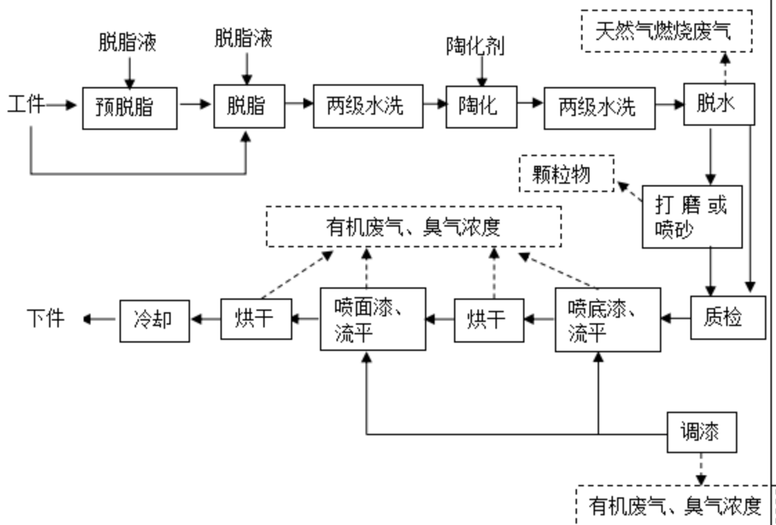
图7 电梯轿厢整体集成系统等喷漆生产工艺流程图
