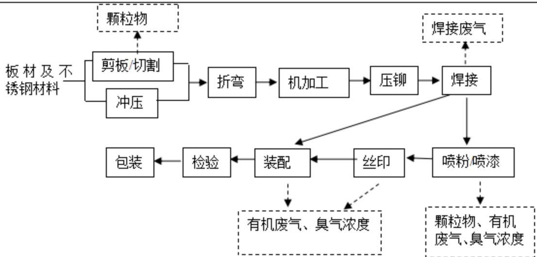
图 5 电梯轿厢等产品生产工艺流程图
