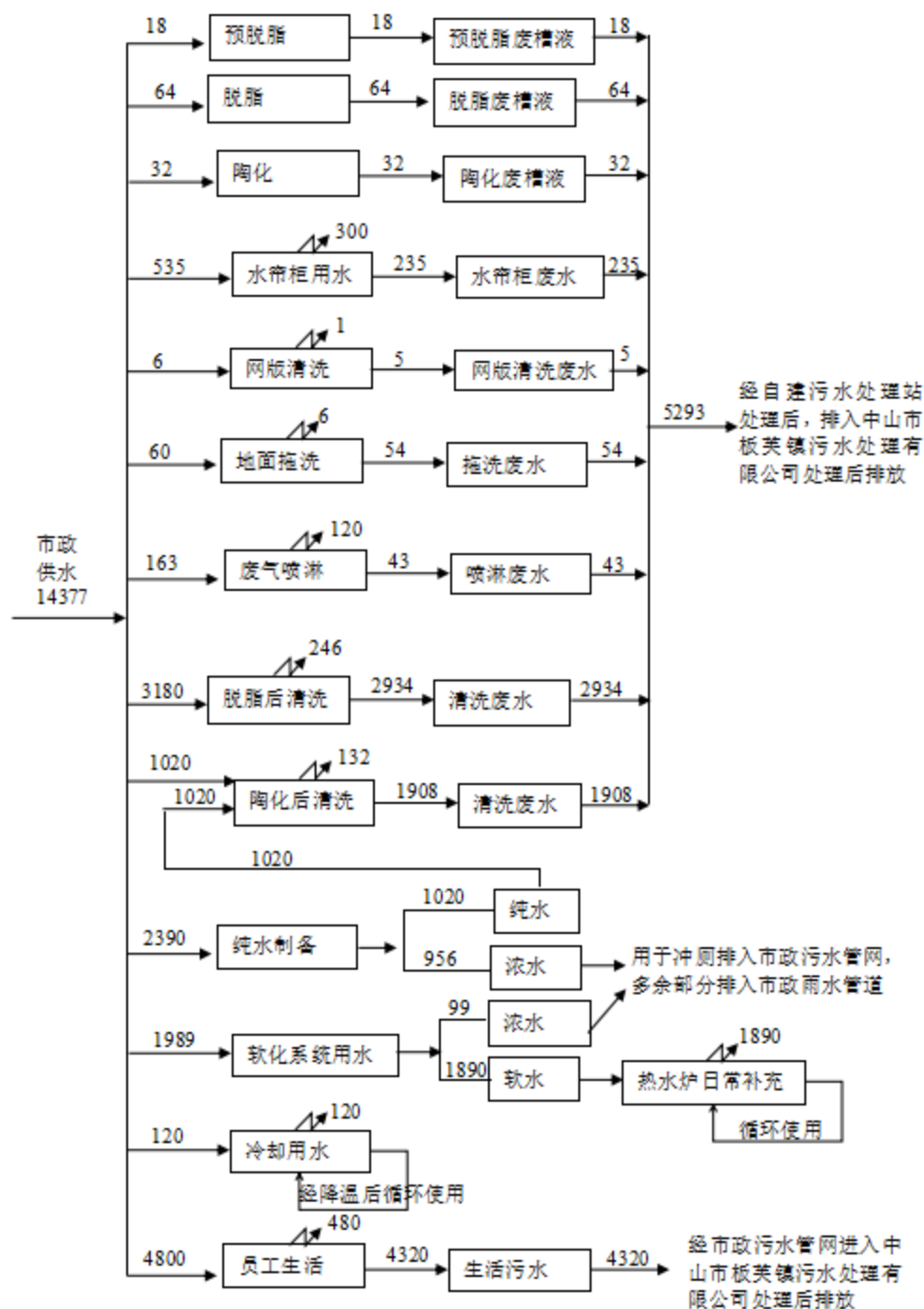
搬迁前水平衡图
