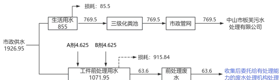
图3 水平衡图 (t/a)
