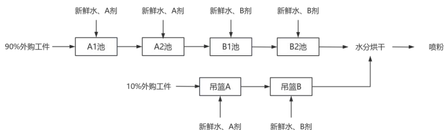
图 2 工件前处理槽体示意图
