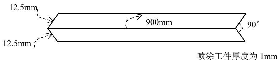
图1 喷涂工件
